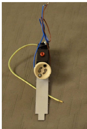
Kit d'adaptation 230V-GU10 pour spot OYSTER (page 118)
